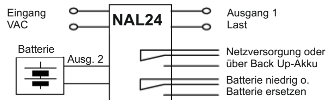
Ausgangs- und Eingangsbeschtaltung
