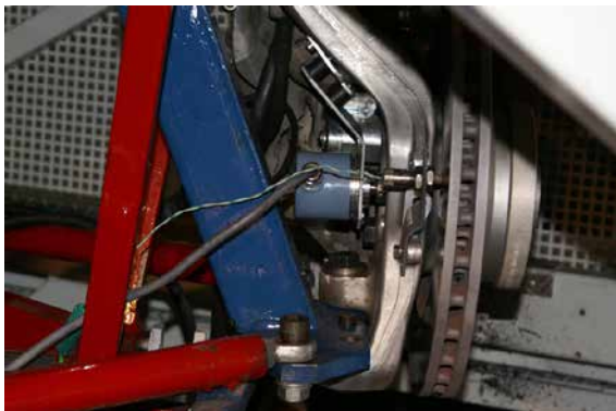
Abbildung 1 Der von Prof. Tiemann entwickelte Viertelfahrzeugprüfstand ist derzeit der einzige weltweit.
